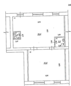
План 1 этажа лит. И2
