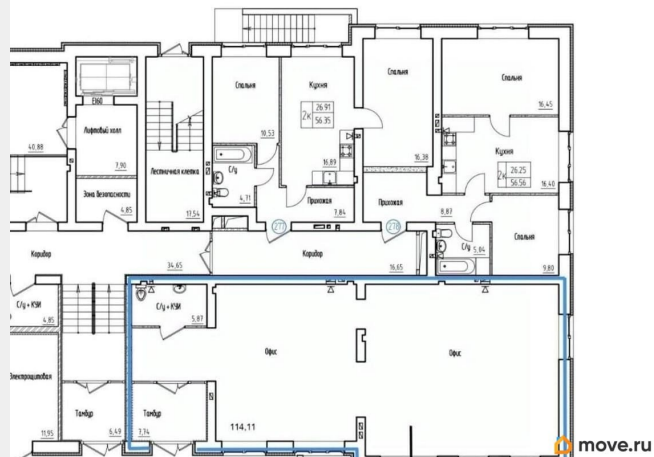
Дом 7. Секция 4. План 1-20 этажа
