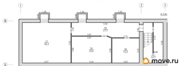
План 1 этажа на отм.-2,300. Лит.А
