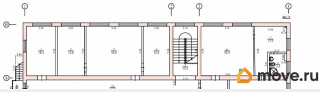
План 2 этажа. Лиг.А
