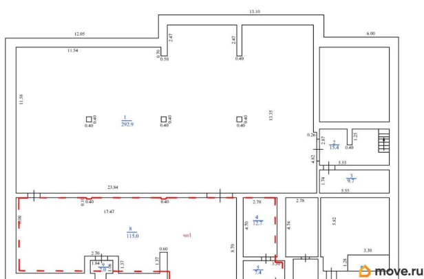
План - 1 этаж
