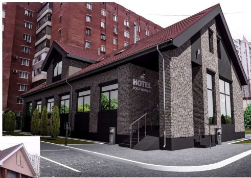
Фотомонтаж 1
